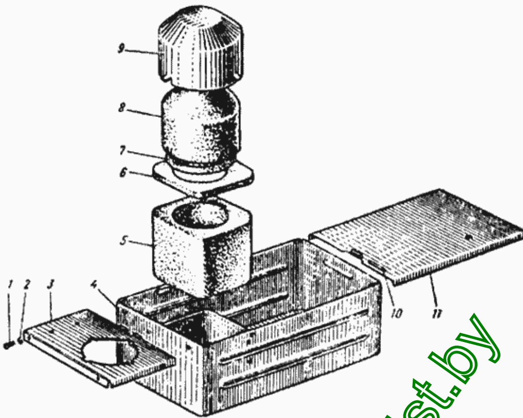
Рис. 56. Инструментальный ящик
